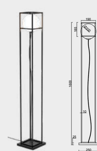
7614 Negro-Black 1LxE27 (no incl)
