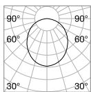
CRI≥90 6W 110° 600lm 3000K
