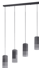
Pendelleuchte · Pendant ↓ 150 cm, ↔ 80,5 cm excl. 4 x E27, max. 28 W
