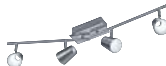
Strahler · Spot ↔ 81,5 x 8 cm, ↓ 20 cm incl. 4 x SMD-LED, 6,5 W 4 x 650 lm, 3.000 K
